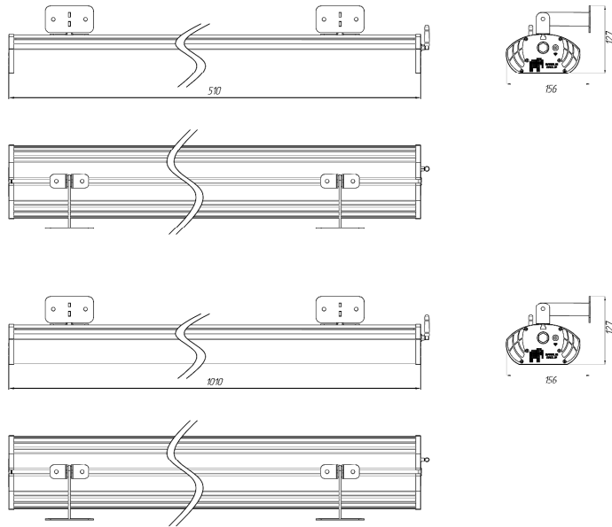
Рисунок 3. Габаритные размеры светильников серии ДСП02. (крепление поворотное)
