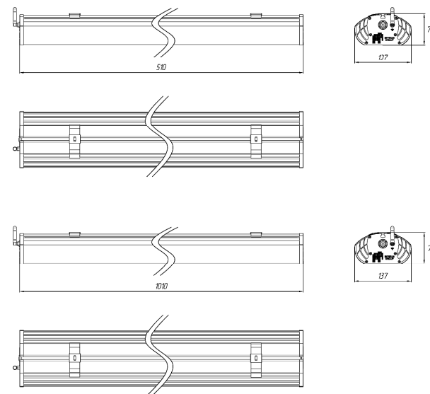
Рисунок 1. Габаритные размеры светильников серии ДСП02.(крепление накладное)
