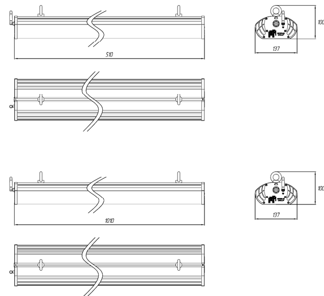
Рисунок 2. Габаритные размеры светильников серии ДСП02. (крепление подвесное)
