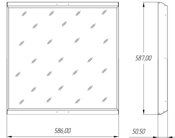
Рисунок 1. Габаритные размеры светильников серии ДПО01
