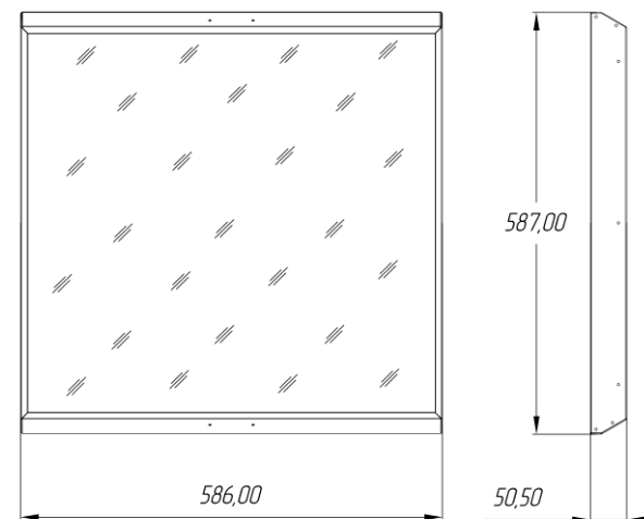
Рисунок 1. Габаритные размеры светильников серии ДПО10
