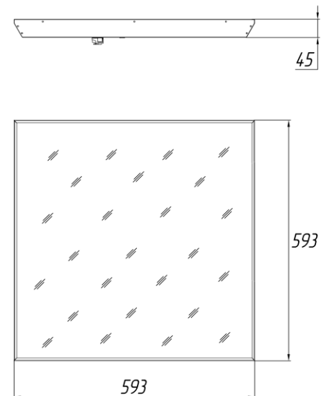
Рисунок 1. Габаритные размеры светильников серии ДВО10
